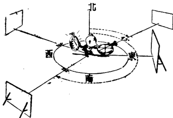
圖4 當喇叭管口旋轉而聽到回聲時，測量羅盤從正北移動的角度，就可算出反射面的方向。
