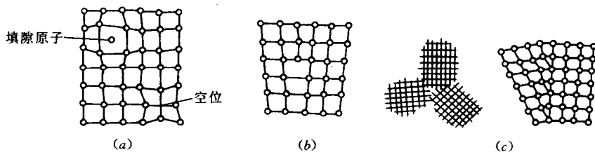
图 1-1 晶格缺陷示意图 (a) 点缺陷；(b) 线缺陷；(c) 面缺陷
