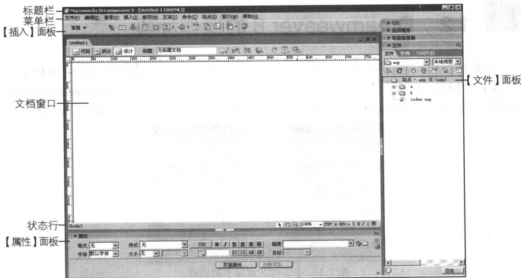
图 1.3 Dreamweaver 8 的界面
