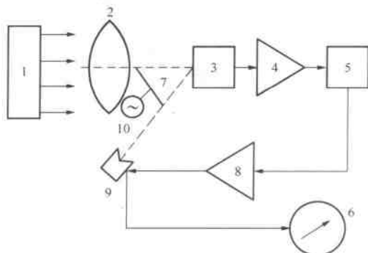
图 1-11 红外测温仪结构
