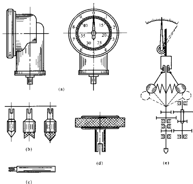
图 1-9 机械式手持转速表及其原理
