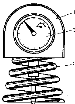
图 1-13 弹簧式振动表结构
