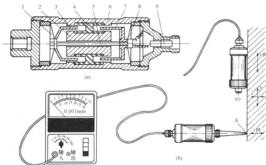
图 1-14 电磁式测振仪
