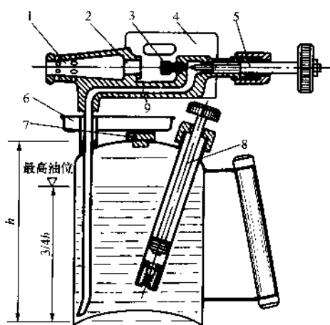
图 1-7 喷灯结构
