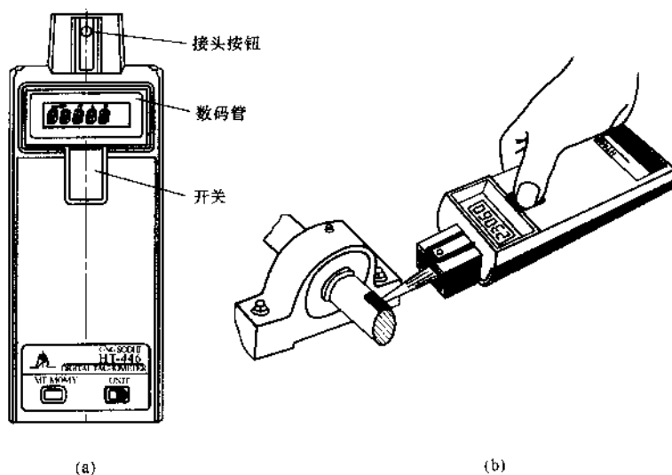
图 1-10 数显式手持转速表
