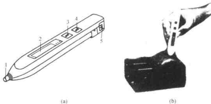
图 1-15 数字式测振笔
