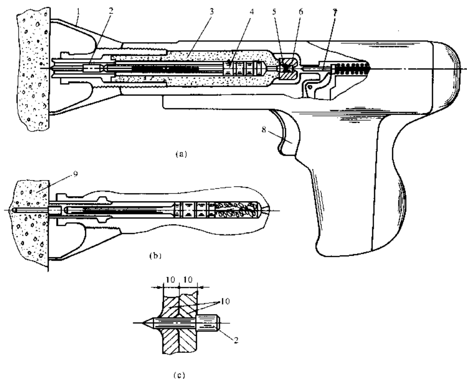
图 1-8 射钉枪结构示意图
