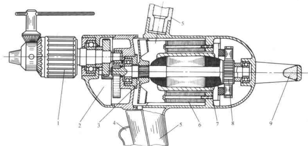
图 1-1 手电钻结构
