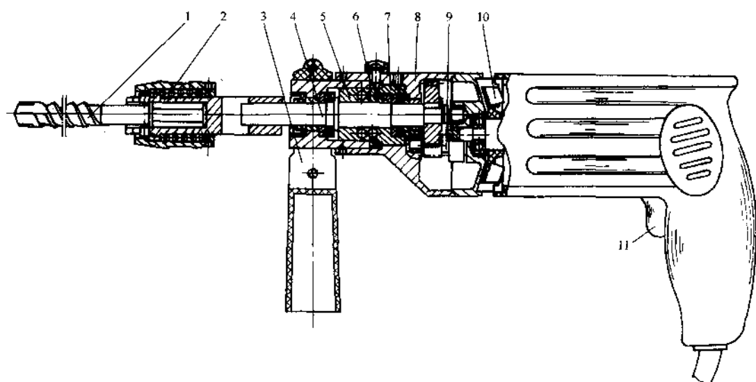
图 1-5 冲击电钻结构
