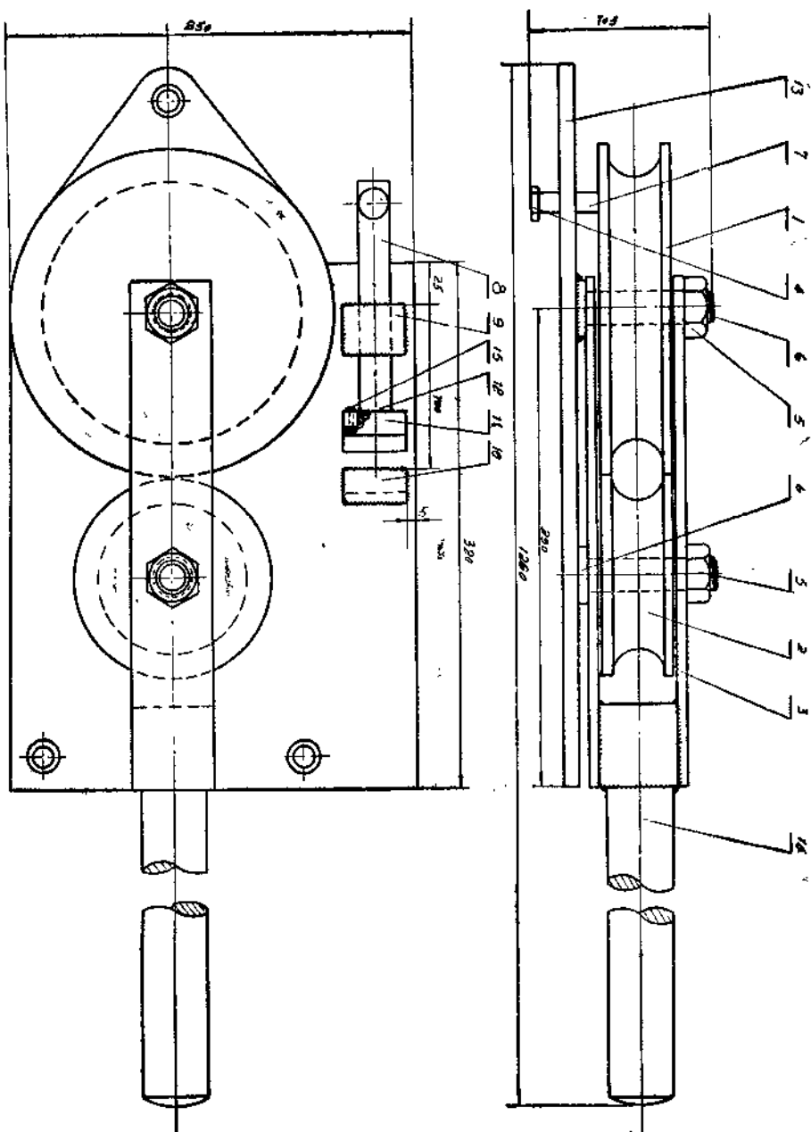
二、手動彎管器施工圖
