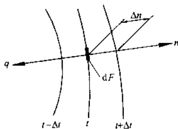
图 14-1 等温面示意图
