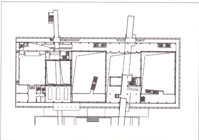
四层平面图
