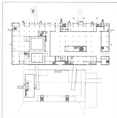
二层平面图
