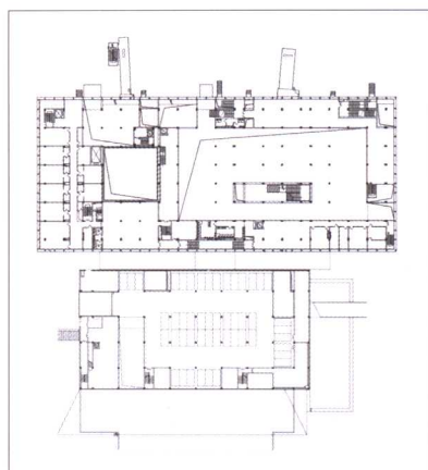
一层平面图
