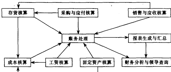
图 1-1 会计核算软件各模块之间的数据传递关系
