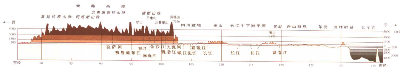
中国地貌海拔剖面示意图。
