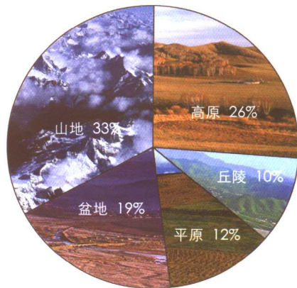
中国地貌比例图。
