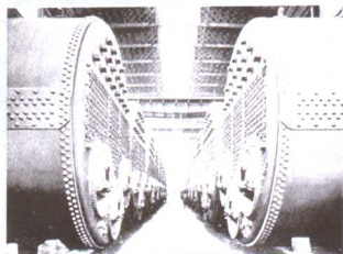
宏伟壮观的锅炉机组 29只锅炉，每只重100吨
