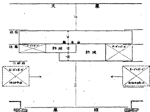
舞台平面圖
