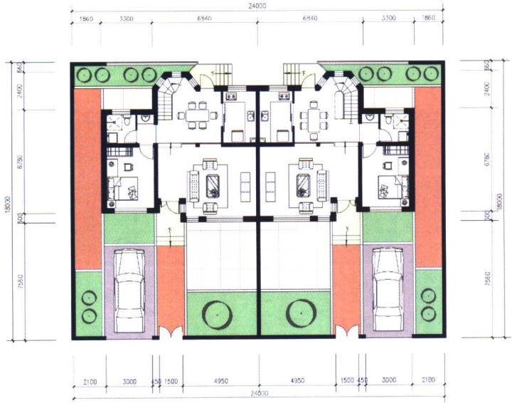
B 户型一层平面
