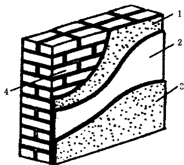
图 1-1 砖墙面抹灰分层示意图
