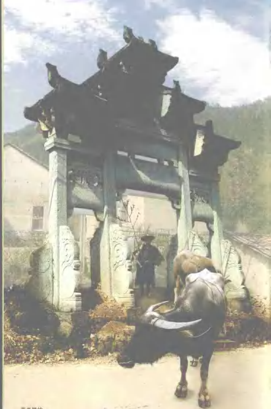
节孝牌坊
