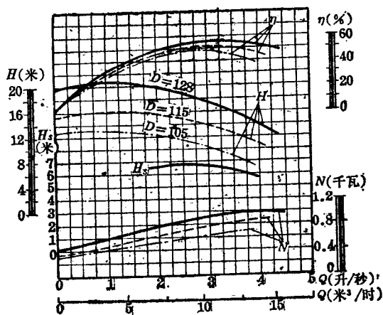
图 1-1 1 1/2 B17型泵性能曲线图
