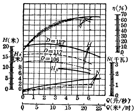
图 1-3 2B19型泵性能曲线图
