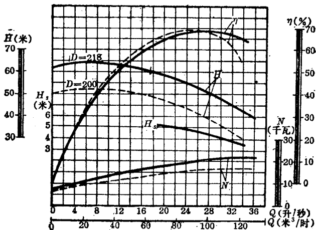
图 1-8 4B54型泵性能曲线图
