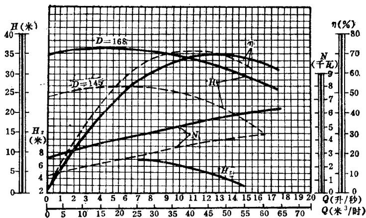
图 1-5 3B33型泵性能曲线图
