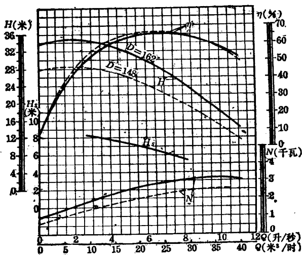
图 1-2 2 B31型泵性能曲线图
