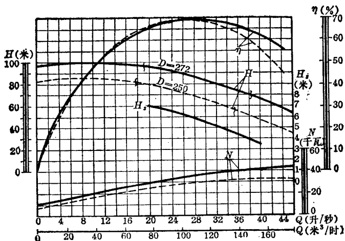
图 1-7 4B91型泵性能曲线图
