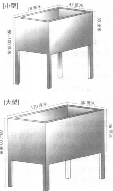
澡盆的规格尺寸
