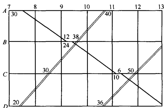
图 1-1-3 小时格列车运行图
