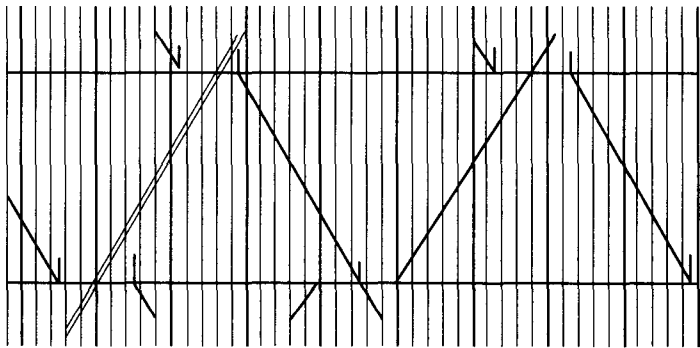
图 1-1-1 二分格列车运行图
