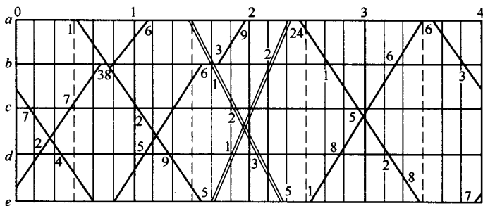
图 1-1-7 单双线列车运行图
