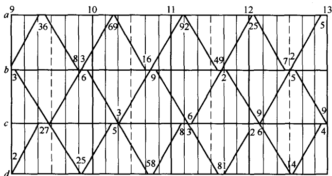
图 1-1-5 单线成对平行列车运行图
