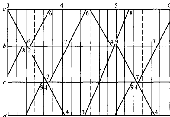
图 1-1-2 十分格列车运行图
