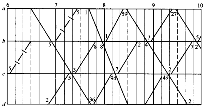
图 1-1-8 单线非平行列车运行图
