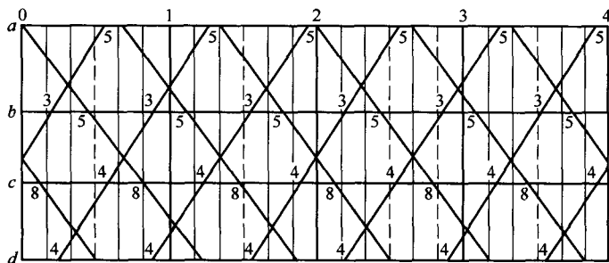
图 1-1-6 双线成对平行列车运行图
