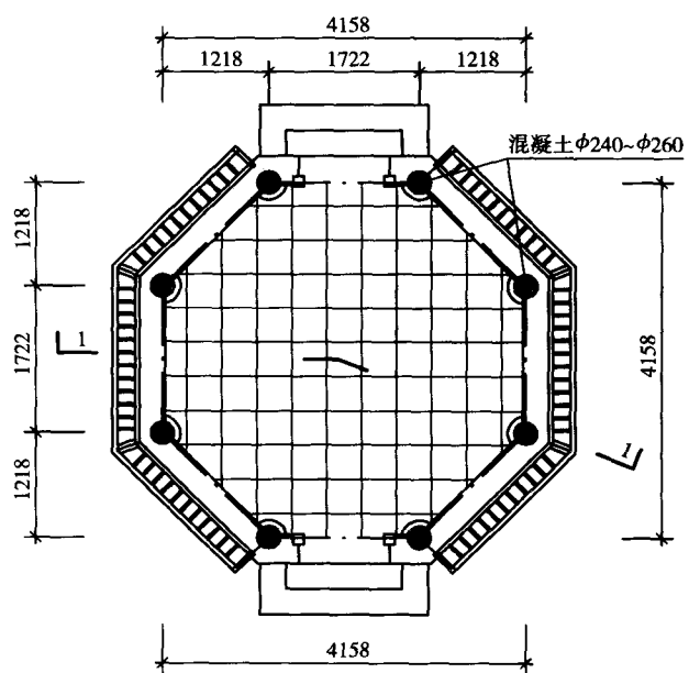
八角重檐亭平面图 1:50
