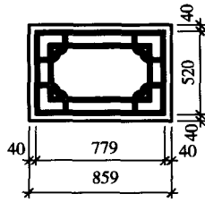
风窗大样 1:25
