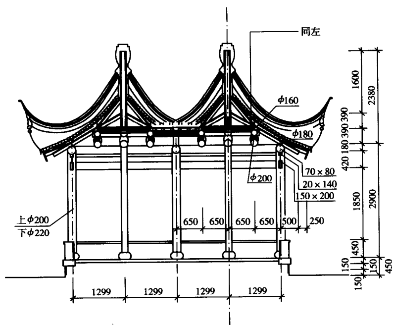
2-2剖面图 1:50
