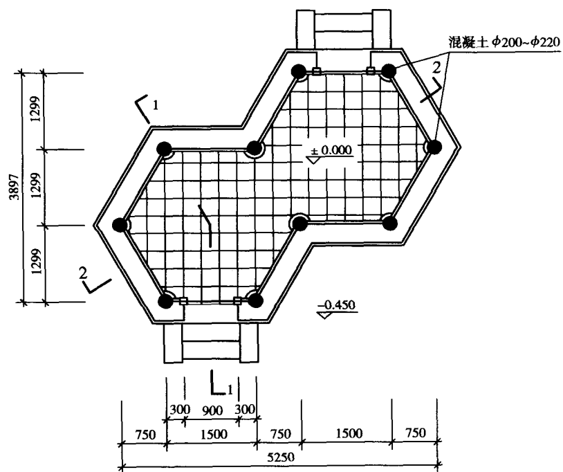
六角套亭平面图 1:50
