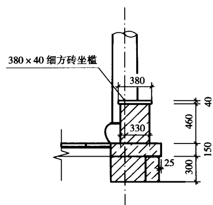
坐槛大样 1:25
