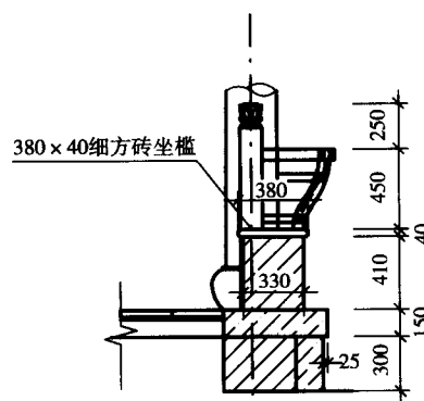
坐槛大样 1:25
