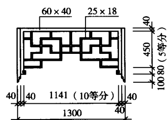
挂落大样 1:25
