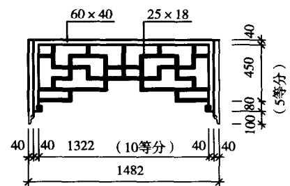
挂落大样 1:25
