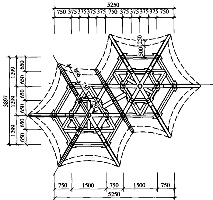
屋架平面图 1:50
