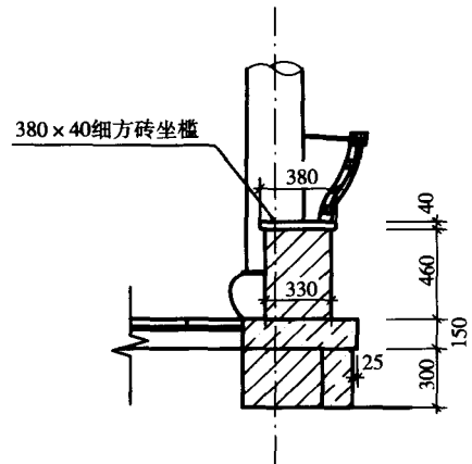
坐槛大样 1:25
