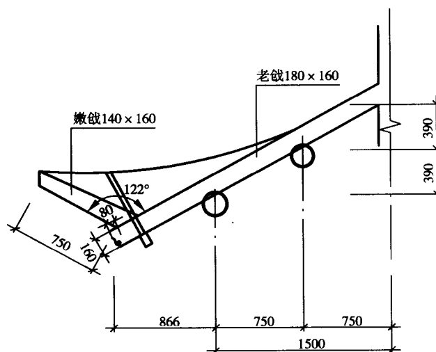
戗角大样 1:25
