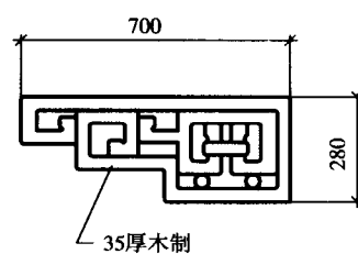
雀替大样
