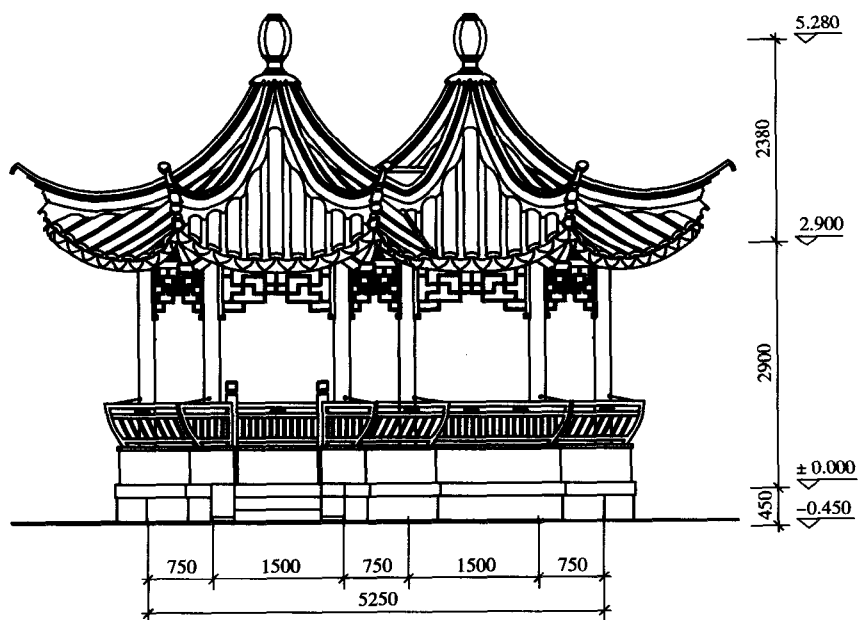
六角套亭立面图 1:50
