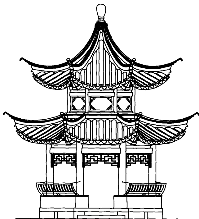
八角重檐亭立面图 1:50
