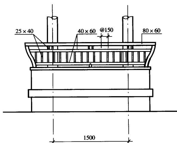
吴王靠大样 1:25
