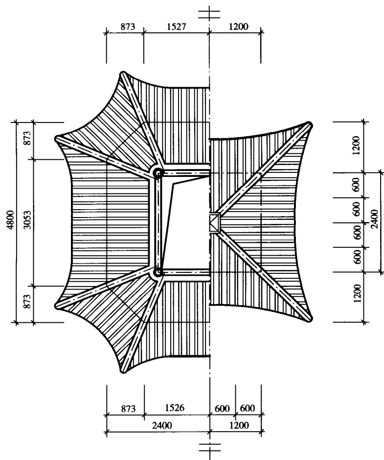
下檐屋面、上檐屋面平面图 1:50
