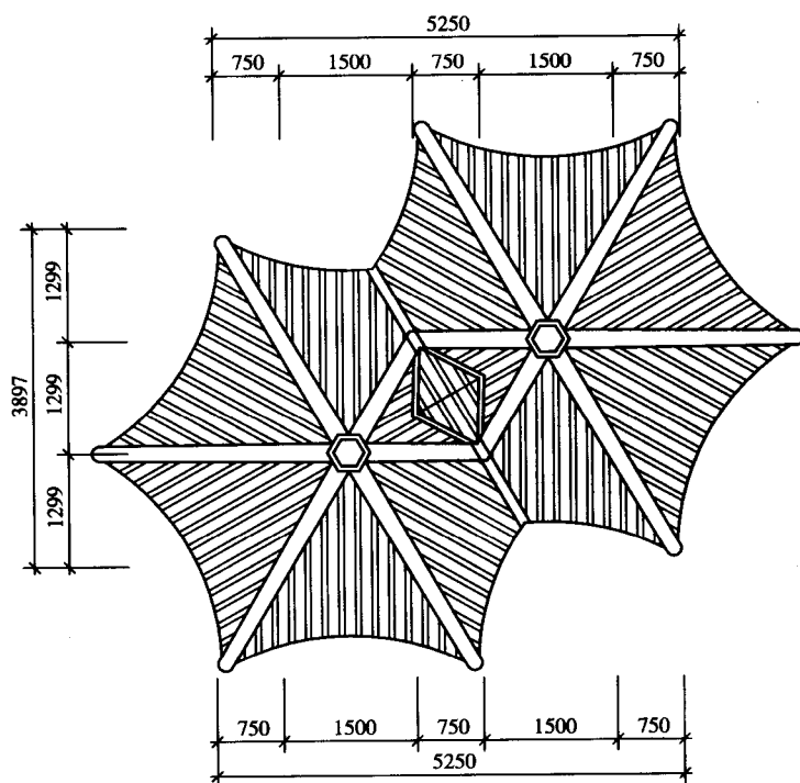
屋面平面图 1:50
