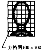
宝顶大样 1:25
