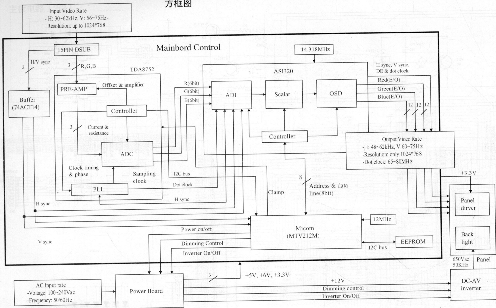
方框图
