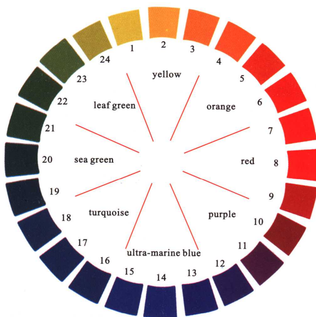
彩图 29 蒙塞尔色相的标定系统
