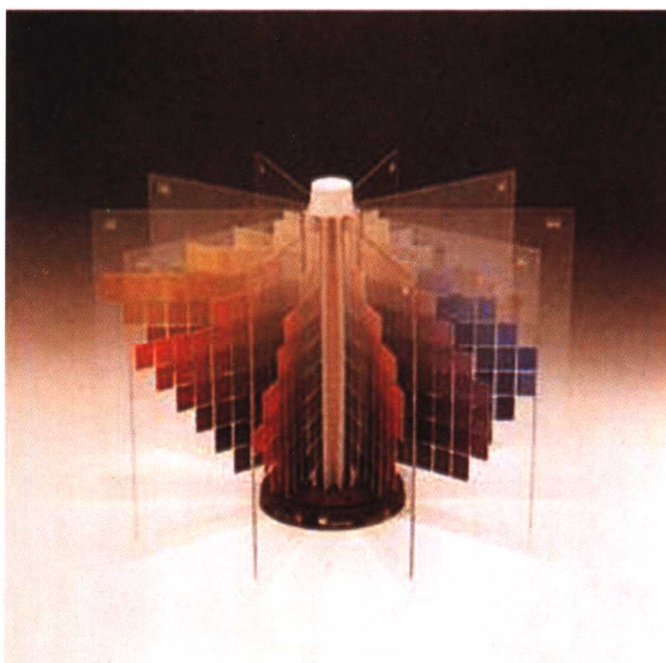
彩图 28 蒙塞尔颜色立体示意图
