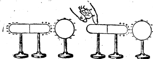
图(1-2) 静电感应。
