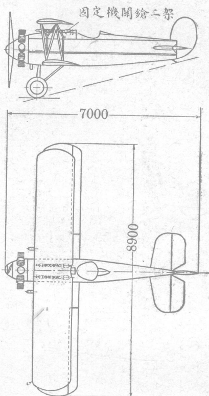
捷克斯拉夫亞維亞 (Avia) 單座戰鬥機設計圖
