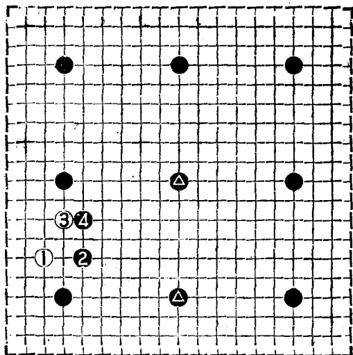
1 谱
