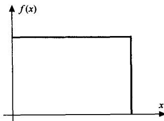
图 1-2 误差的均匀分布曲线
