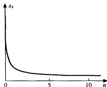
图 1-5 s_{\bar{x}} 与测量次数 n 的关系
