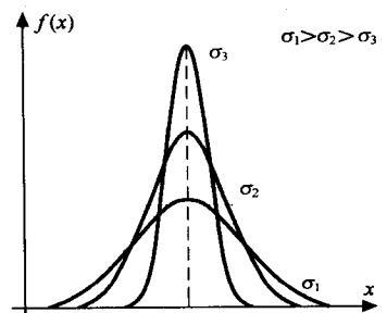
图 1-4 标准差与数据离散程度的关系示意图
