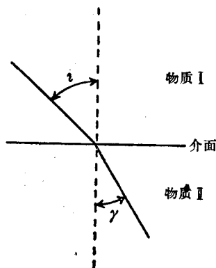
图2 光的折射
