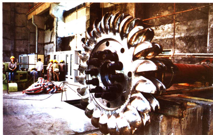
白水河二级 电厂的水轮机组
