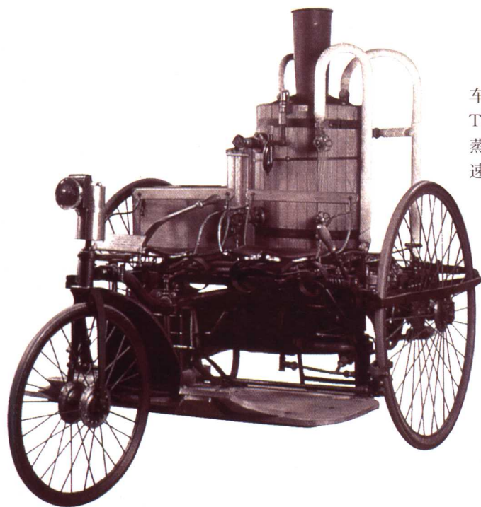
斯科特(Scotte)蒸汽载客车 1892 2 气缸, 排量 1986mL, 最高速度12km/h。
