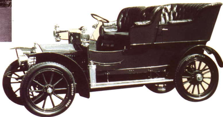
劳斯莱斯(Rolls Royce) Bicylinder 1904 劳斯莱斯在汽车史上是个不能 忽视的品牌, 这辆1904年的劳斯莱斯有 两个气缸, 排量为1809mL, 功率7.5kW (10HP), 最高时速可达到60公里。
