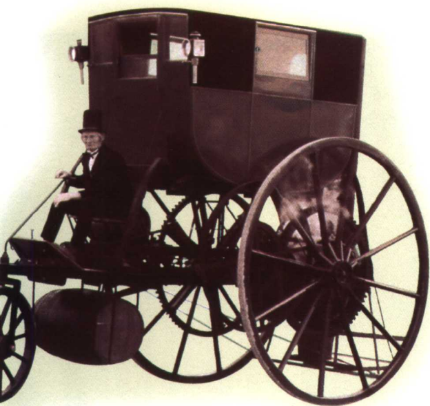
斯雷维斯克蒸汽汽车 (Threvithick's London Stream Carriage) 1803 这辆重心很高的蒸汽汽车 采用单缸设计，功率为3 马力，每小时最快行驶 13 公里。
