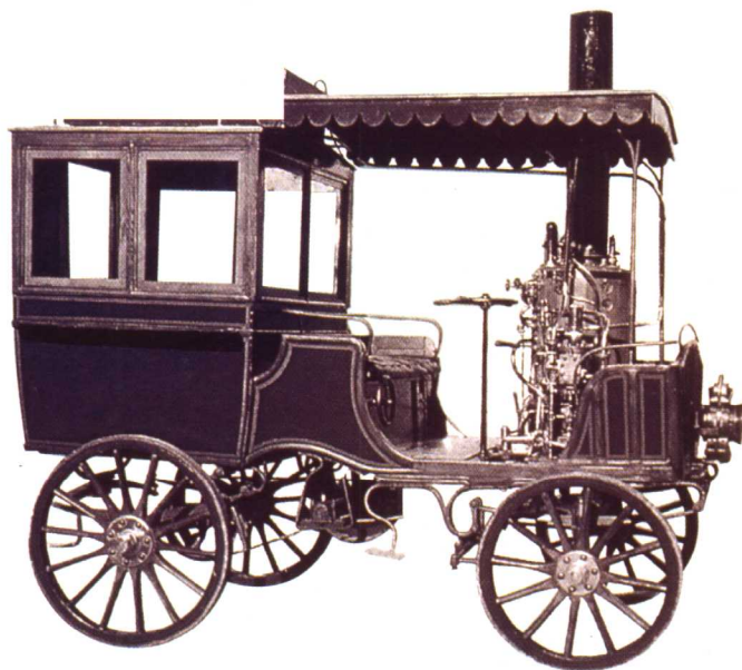
斯科特(Scotte)蒸汽载客车 1892 2 气缸, 排量 1986mL, 最高速度12km/h。
