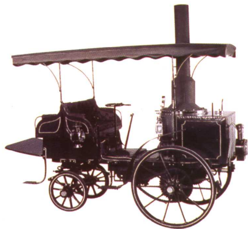
德迪恩-博顿“狗拉小车”(De Dion- Bouton dog-cart) 1885 这辆有着奇 怪名字的蒸汽机车最高时速可达40公里。
