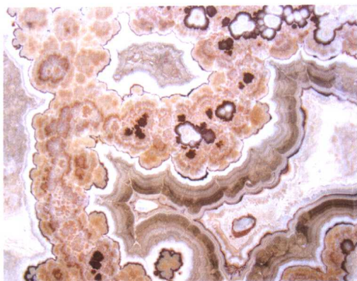
昆仑彩石
