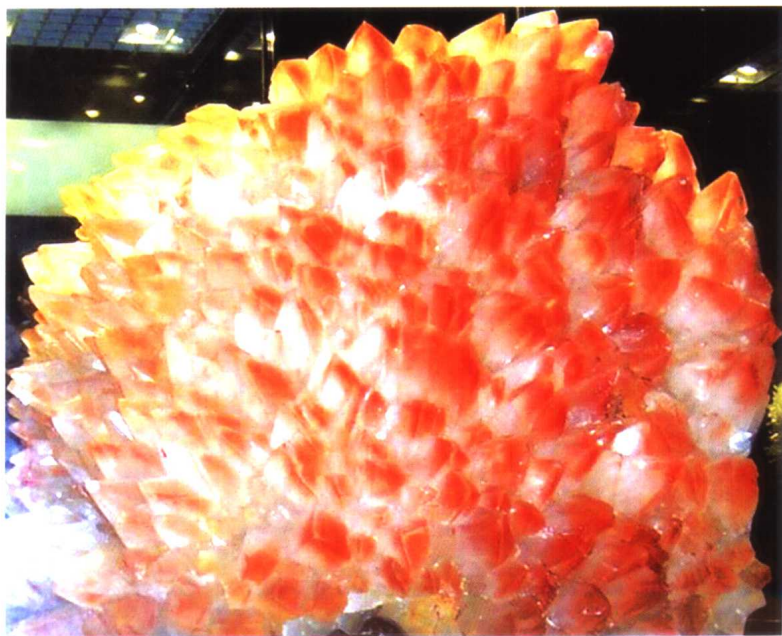
方解石晶簇
