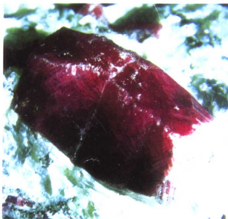
刚玉
