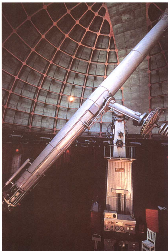
利克天文台的91厘米克拉克折射望远镜是世界上第二大折射望远镜。
