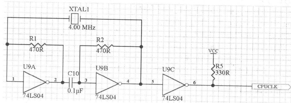
图 1-2 CPUCLK 方块图的原理图子图
