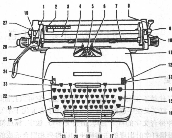
图 1. 打字机主要部件及名称
