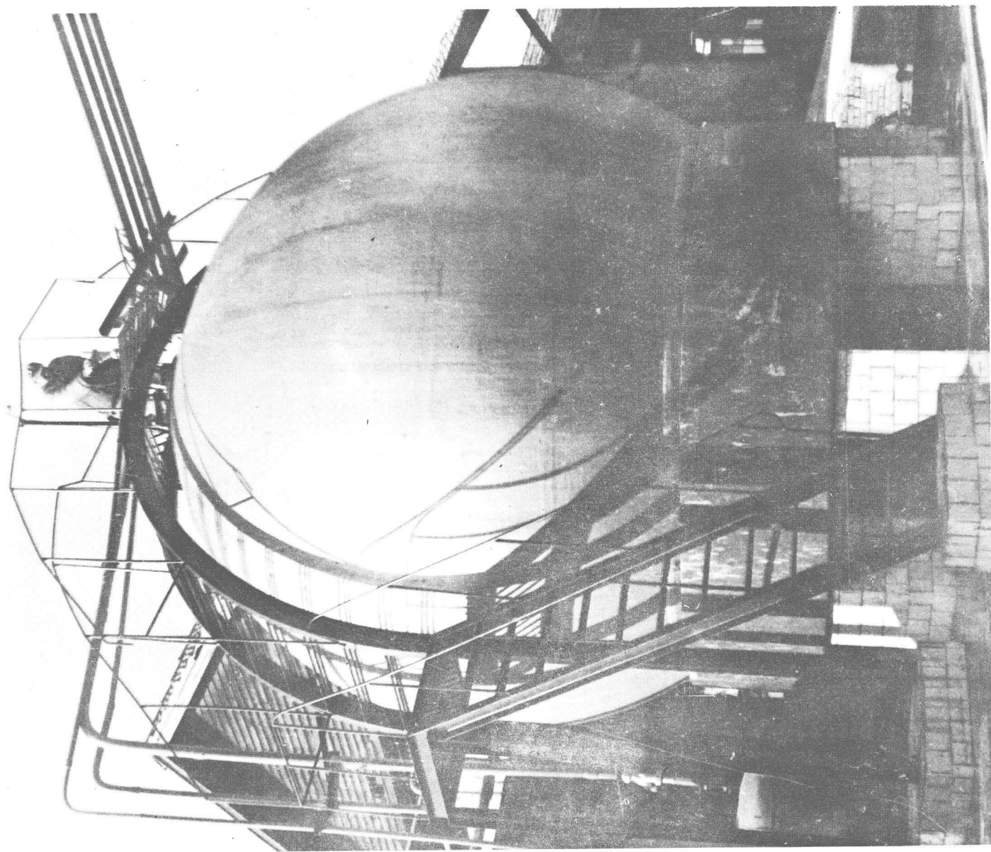
75 米 3 球形盐酸贮槽 (衢州化工厂)
