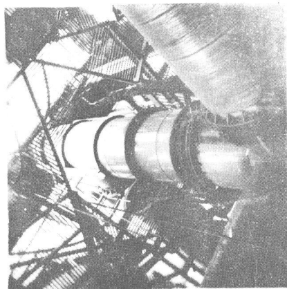
二氧化硫管道 (衢州化工厂) \phi 1000 , \delta 15 毫米。硬聚氯乙烯
