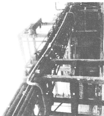
硝酸管道 (南京化肥厂) D g 100, L300000 毫米。硬聚氯乙烯 介质: 45% 硝酸。P3 公斤/厘米 2 自 1961 年使用至 1972 年, 现仍继续 生产
