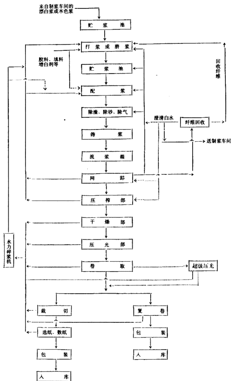
纸张生产流程简图
