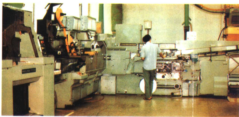
引进英国莫林公司的超九五机组,每分钟卷制6500支
