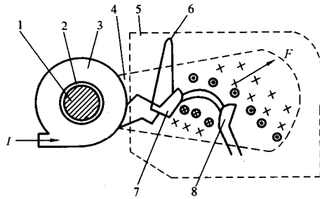
图 1-5 磁吹式灭弧装置
