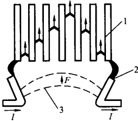
图 1-4 栅片灭弧示意图
