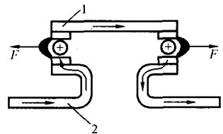
图 1-3 桥式触头灭弧原理 1—动触头; 2—静触头
