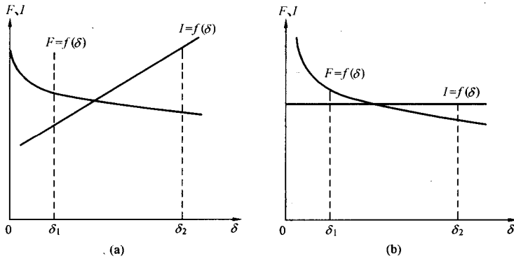
图 1-8 吸力特性
