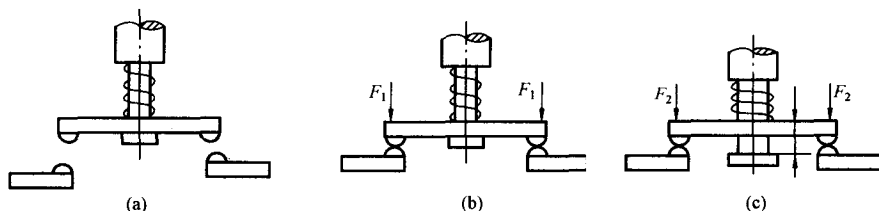
图 1-2 桥式触头闭合过程位置示意图
