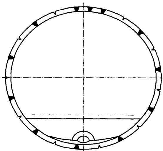
图 B.4 内弧面浇注弧形块隧道
