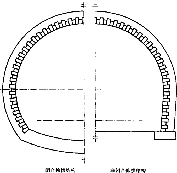
图 B.1 砖石结构隧道
