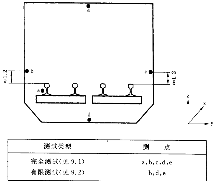
图 1 根据测试类型布置隧道横断面测点
