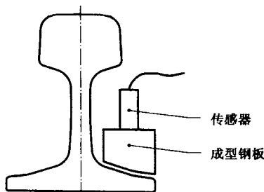
图 2 钢轨底部的测点
