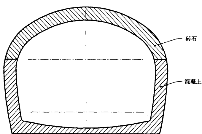
图 B.3 混合砖石结构隧道
