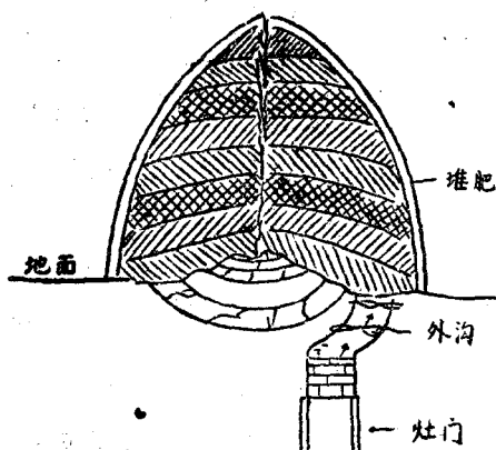
盘龙式堆肥縱剖面图
