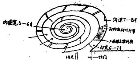
盘龙式堆肥縱剖面图
