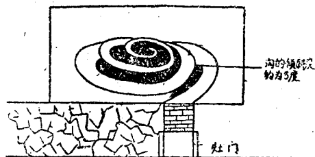
盘龙式堆肥沟道立体图
