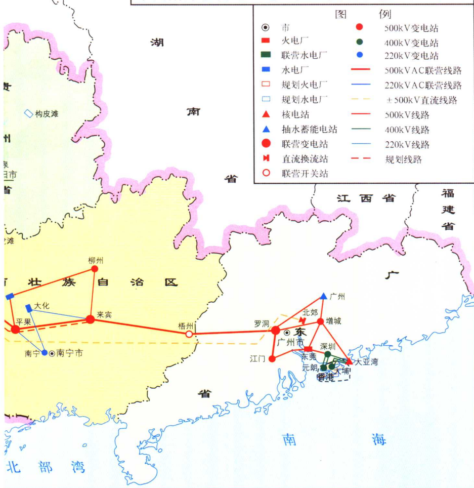
中国南方联营电网地理位置接线示意图(1993年)
