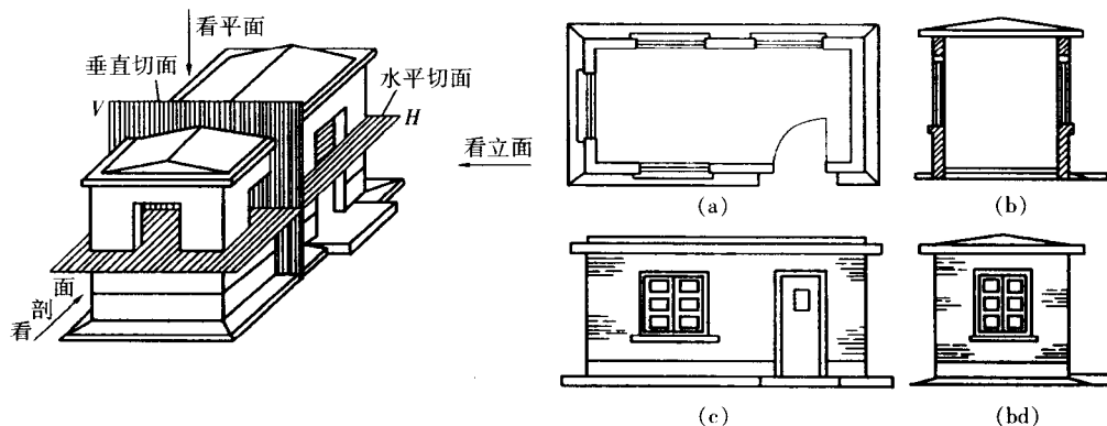
图 1-9 房屋的剖切视图
