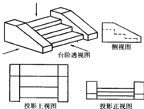
图 1-7 物体的投影视图
