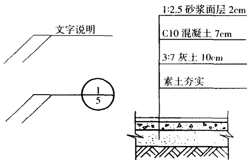
图1-20 引出线
