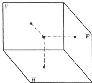
图 1-4 点的投影
