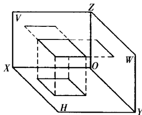
图 1-6 面的投影
