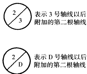
图 1-13 附加轴线标志法
