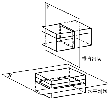
图 1-8 平面剖切物体图示
