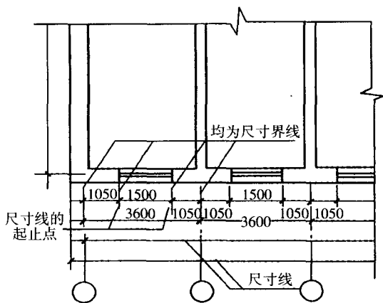
图1-17 尺寸线标法
