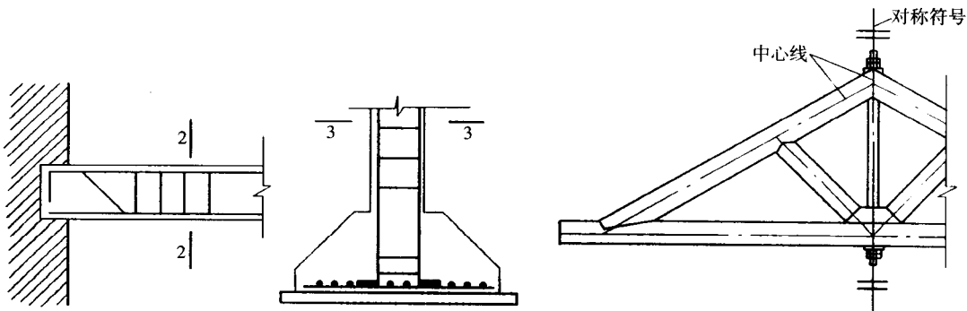
图 1-15 剖视号的标志方法
