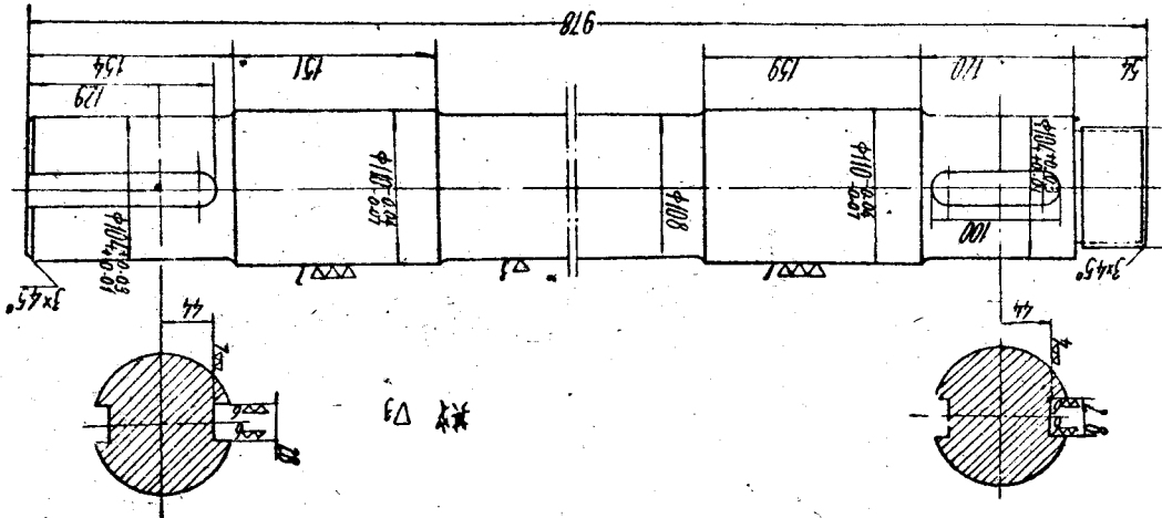
10-6 轴45号钢1件
