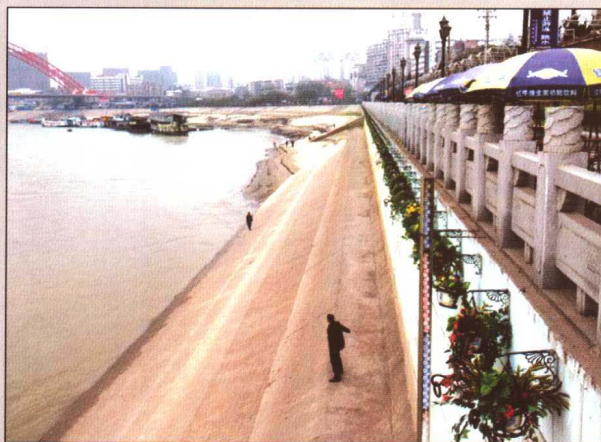
加固后的武汉市龙王庙城市堤防工程
