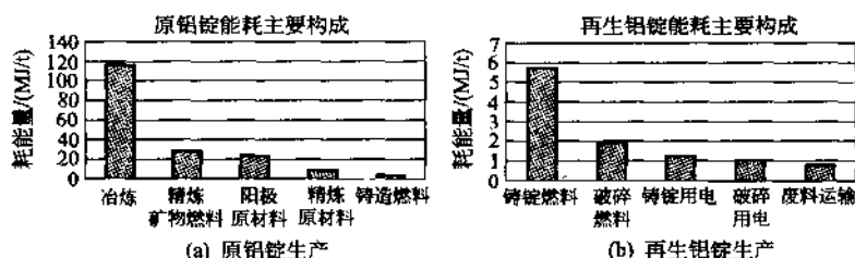
图 1-5 原铝和再生铝生产的能量消耗分布及消耗量
