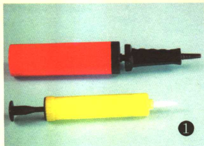
图①上为双向打气筒，推下去和拉回来都会充气；下为单向打气筒，只有先拉出，推下时才能充气。
