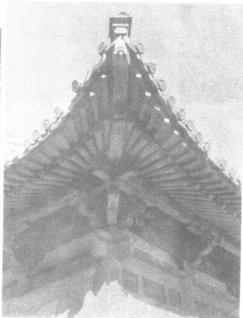
(乙) 觀音殿轉角鋪作
