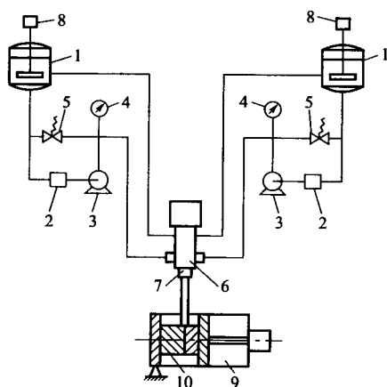
图 1-3 反应注射成型
