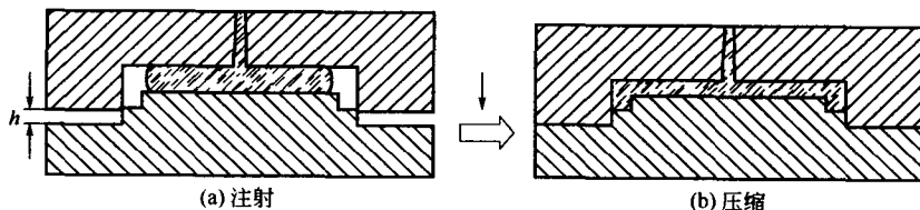
图 1-4 注塑-压缩成型原理示意图
