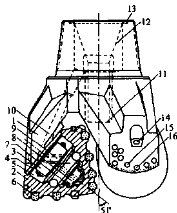
图 2-6-3 牙轮钻头结构
