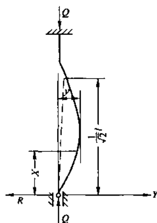
图 2-6-4 钻杆受压的挠曲线
