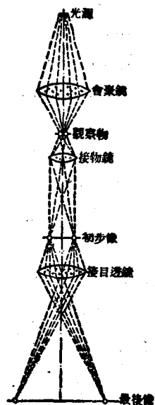
圖3 投影式光學顯微鏡中光線的進路。
