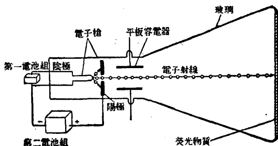
圖 7 電子射線管。
