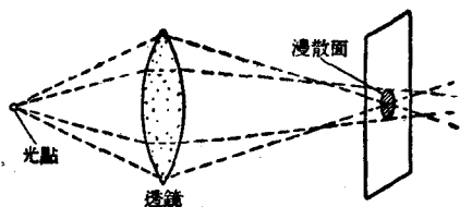
圖4 球形像差。
