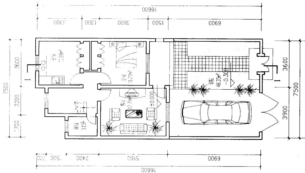
底层平面图
