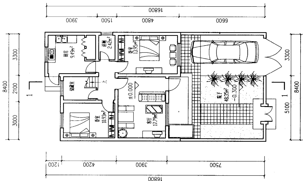
底层平面图
