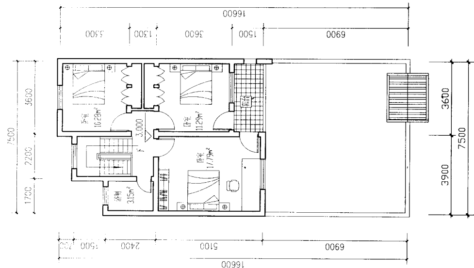
二层平面图
