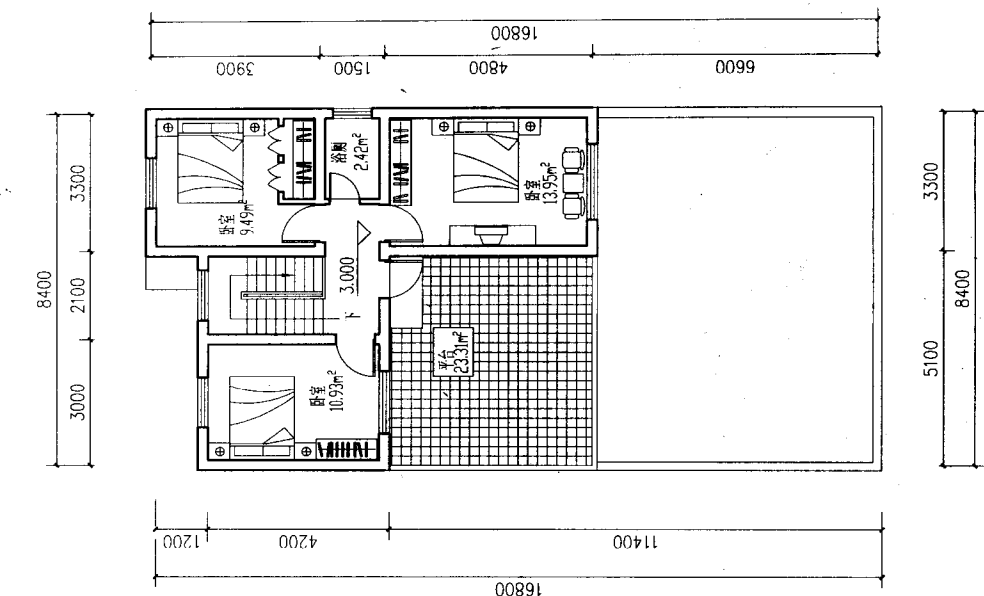
二层平面图
