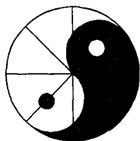
太极图
