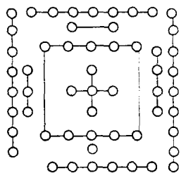
河图
