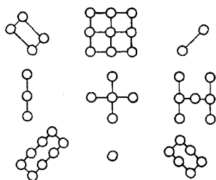
洛书
