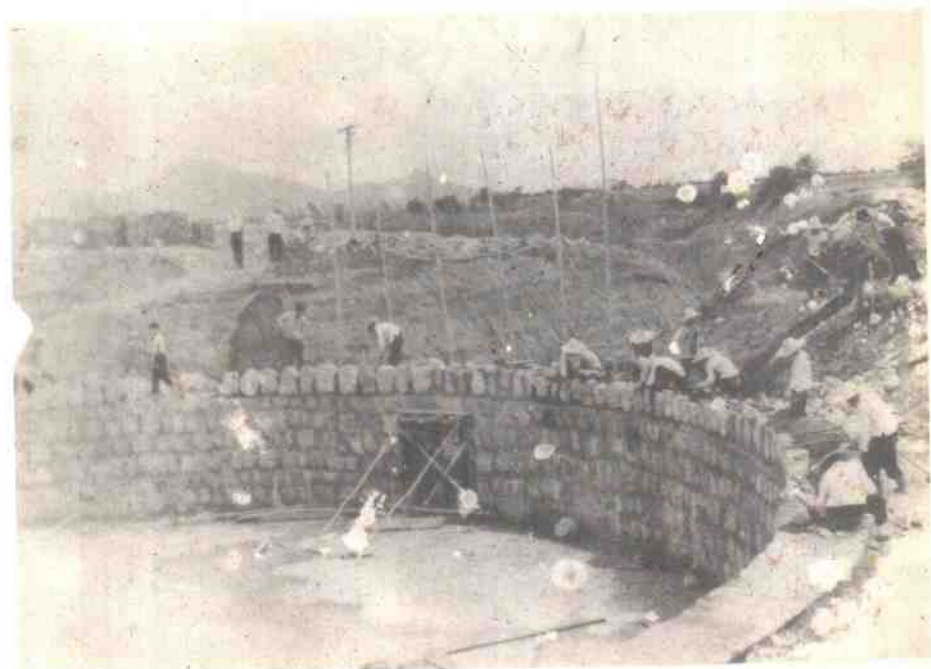
覆土油罐土石方工程
